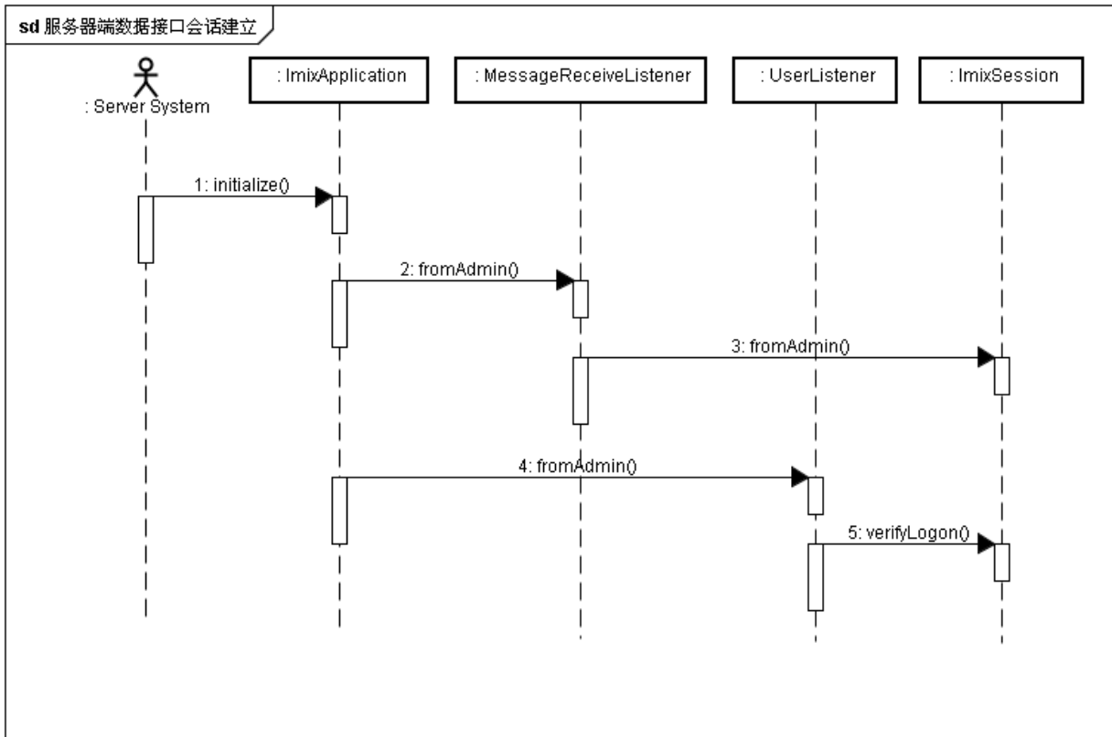
图5 Server 端数据接口建立时序图
