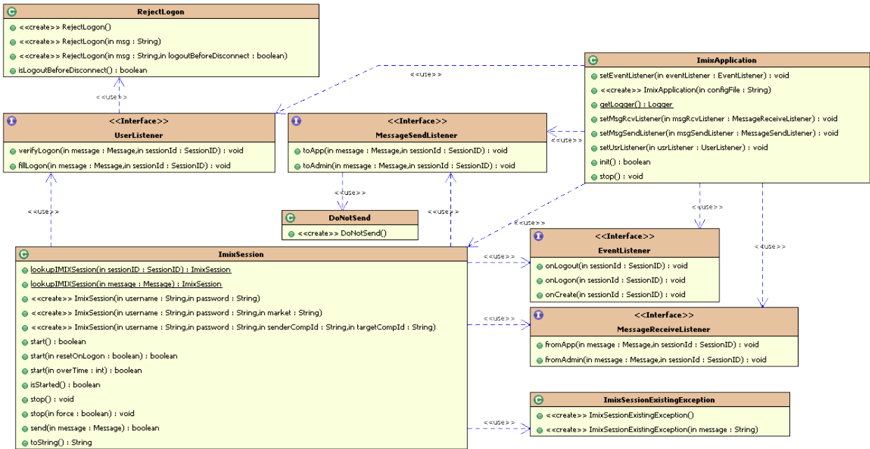
图3 Server 部分主要类图
