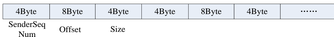
图16 Header 文件结构
