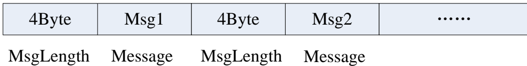
图20 Queue 文件结构
