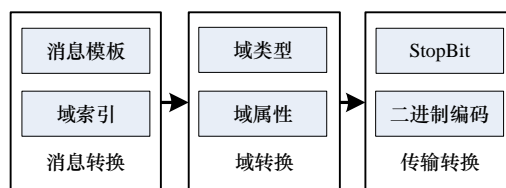
图11 数据传输压缩接口流程
