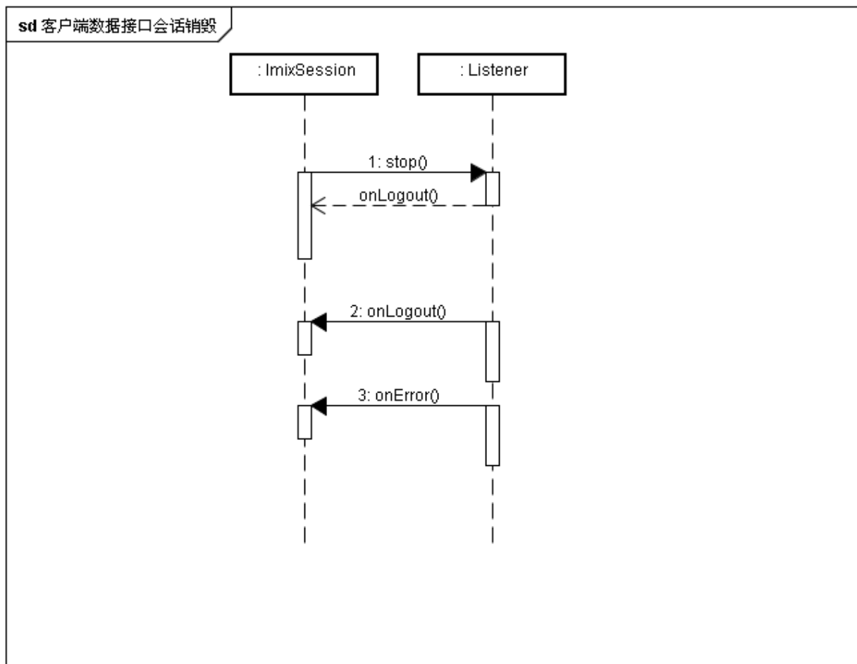
图6 Client 端数据接口会话销毁时序图
