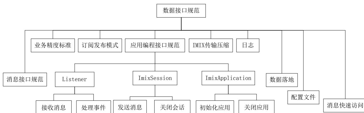
图1 数据接口整体结构框图
