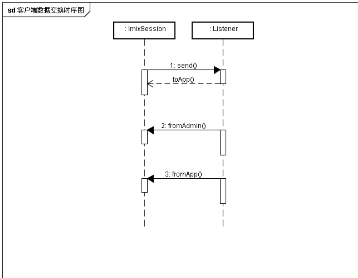
图8 Client 端数据交换时序图
