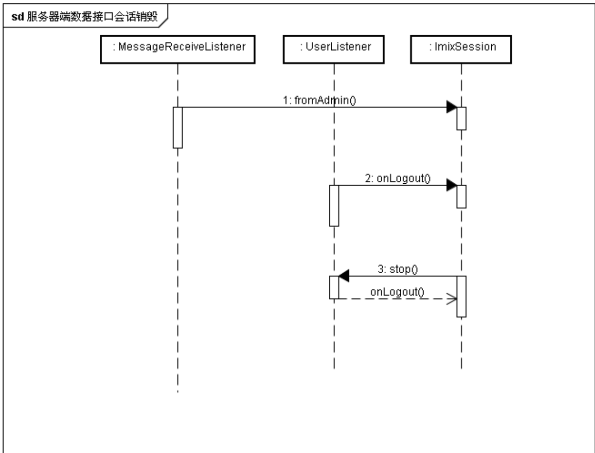
图7 Server 端数据接口会话销毁时序图
