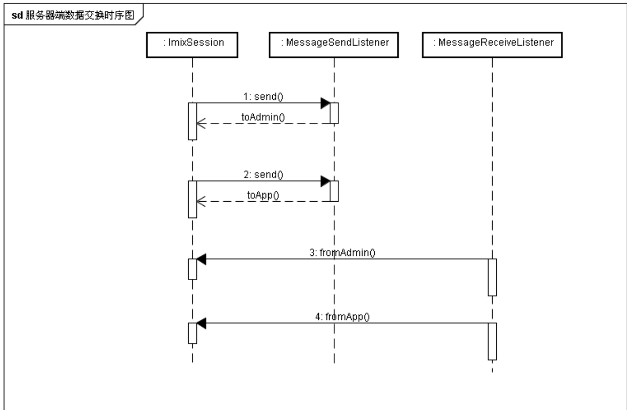
图9 Server 端数据交换时序图
