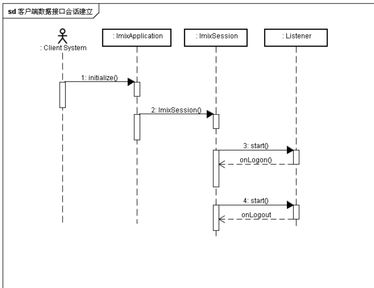
图4 Client 端数据接口建立时序图
