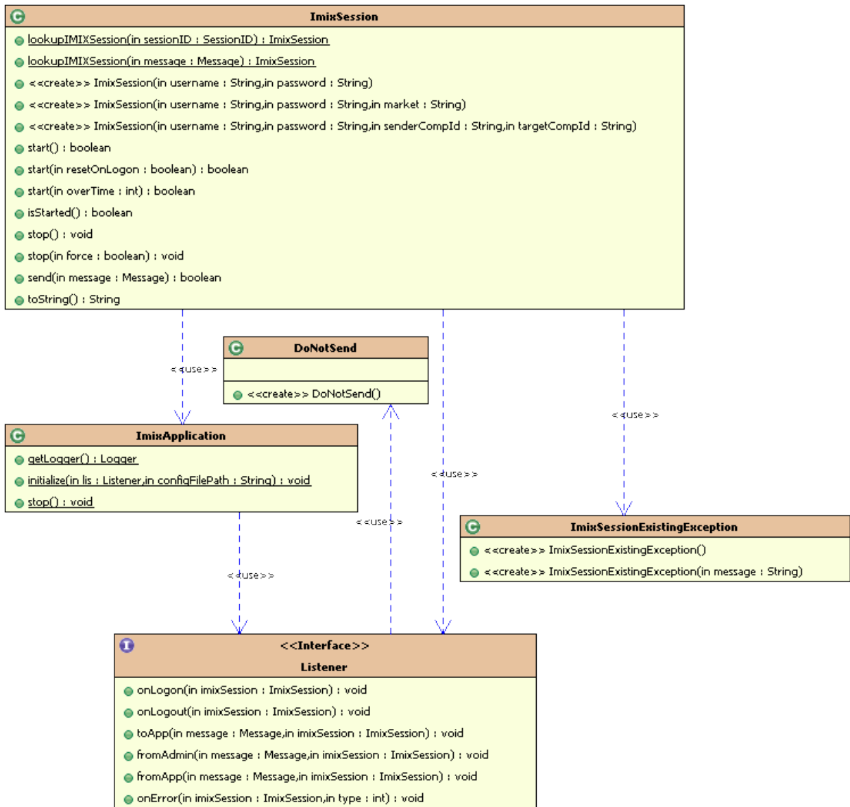
图2 Client 部分主要类图
