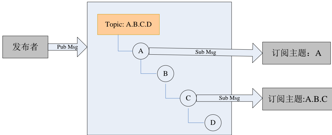
图22 分层次主题命名
