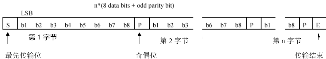
图9 标准帧
