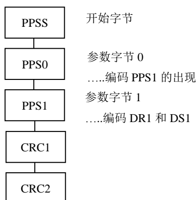
图46 协议和参数选择请求
