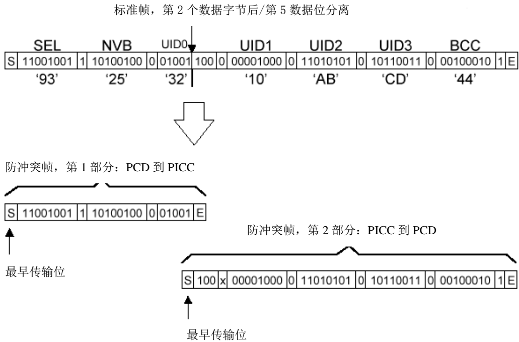
图11 面向位的防冲突帧的位组织结构和传输，分离字节 对于SPLIT BYTE，PCD应忽略第二部分的第一个奇偶校验位。
