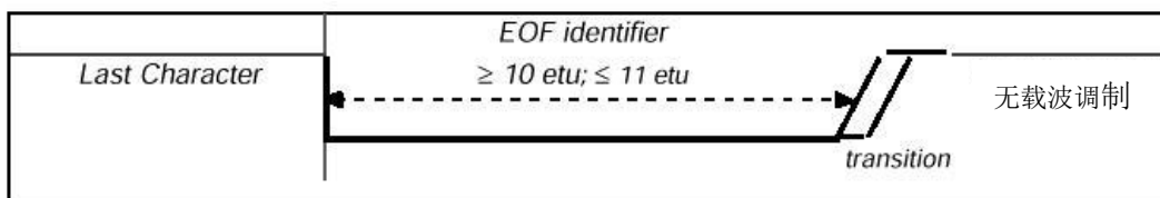
图21 EOF 标识符
