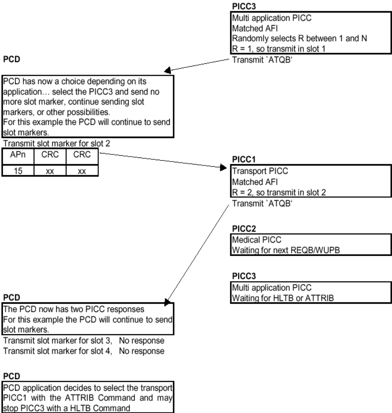
图 E.1 Type B 防冲突序列举例 1
