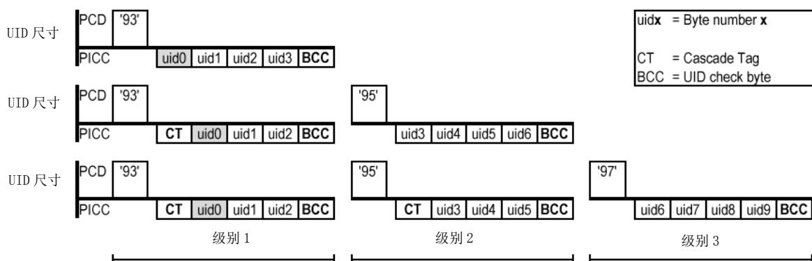
图17 串联级别的使用
