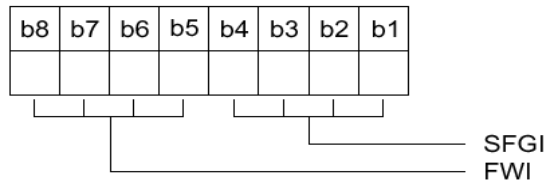
图44 接口字节 TB (1) 的编码
