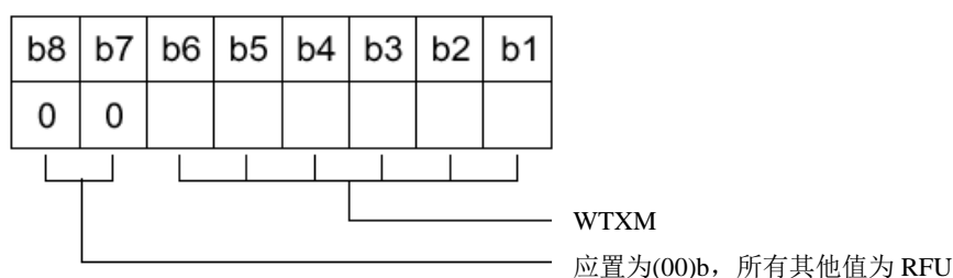
图58 S(WTX) 响应的 INF 域编码
