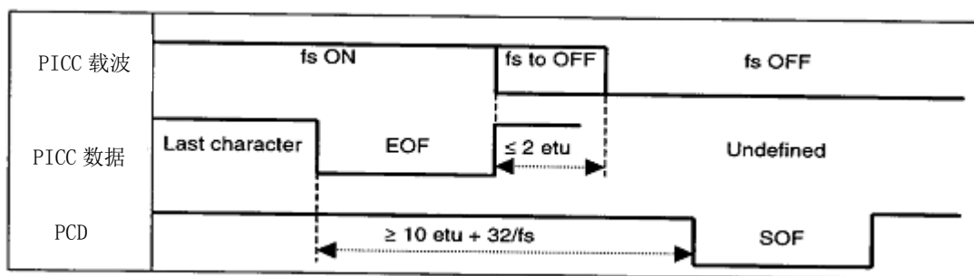
图23 PICC 到 PCD 的 SOF
