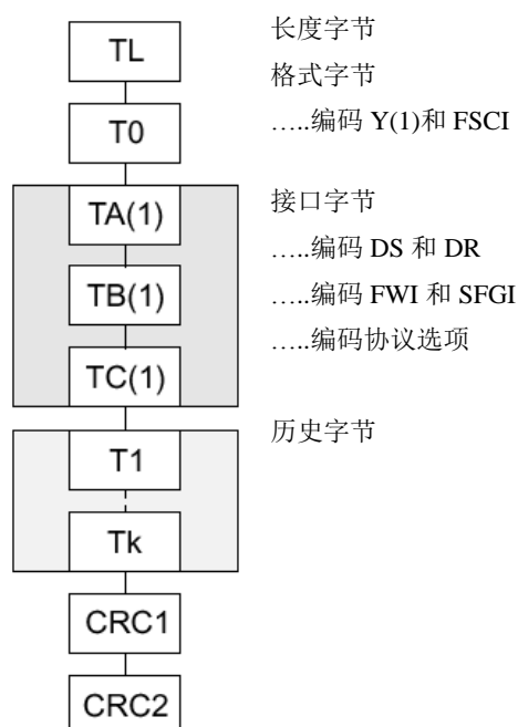
图41 ATS 的结构
