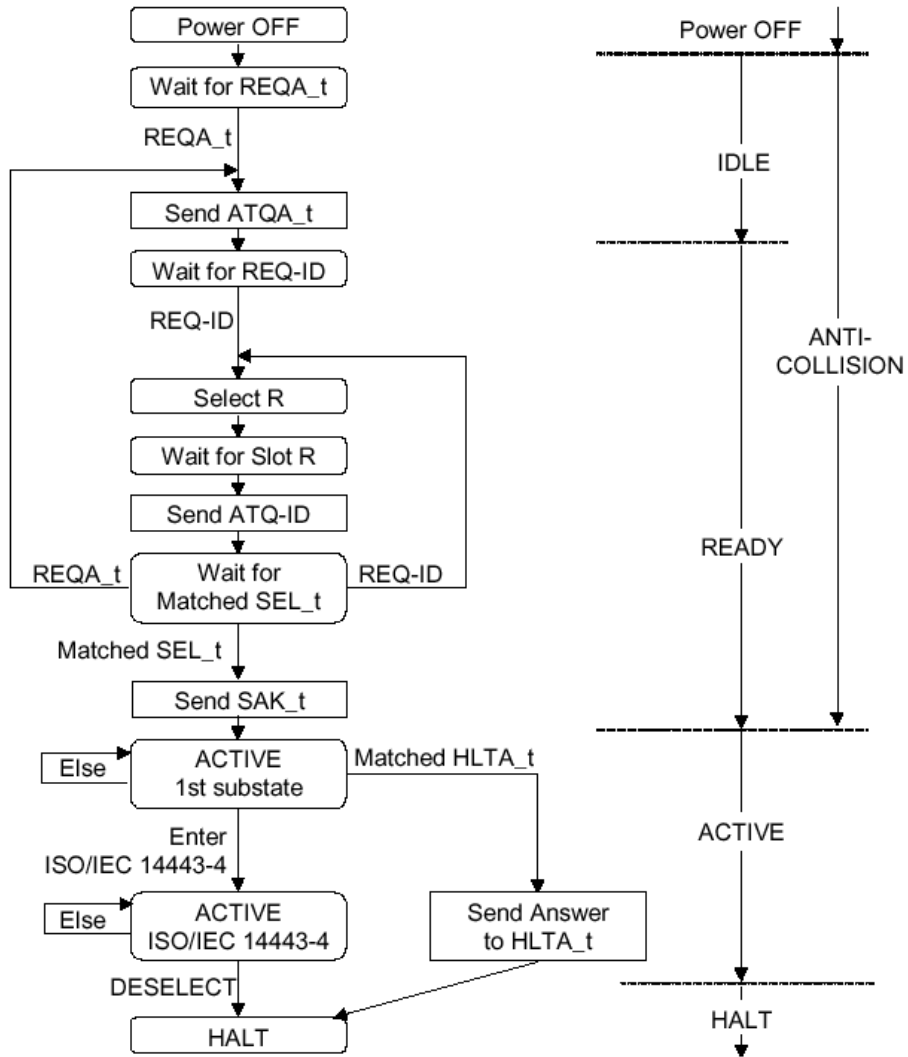
图 D. 2 时间槽-Type A 防冲突流程图
