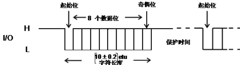
图10 字符帧
