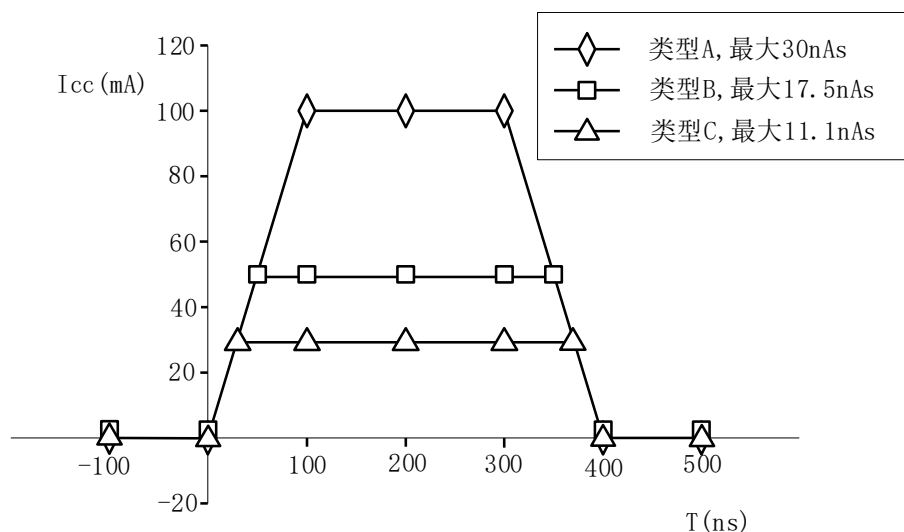
图5 最大电流脉冲包络
