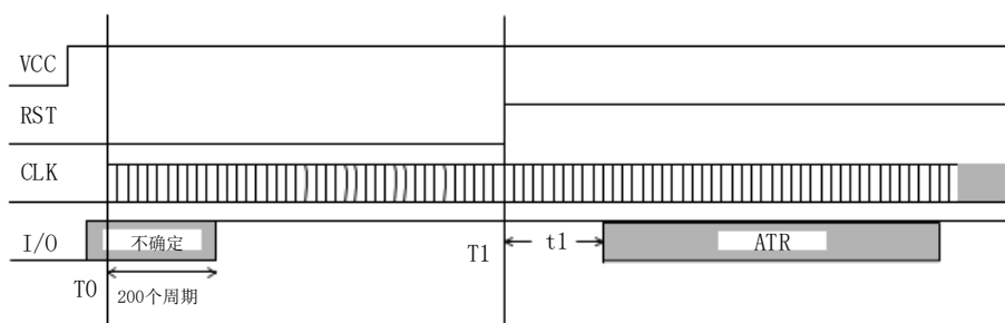
图7 冷复位时序
