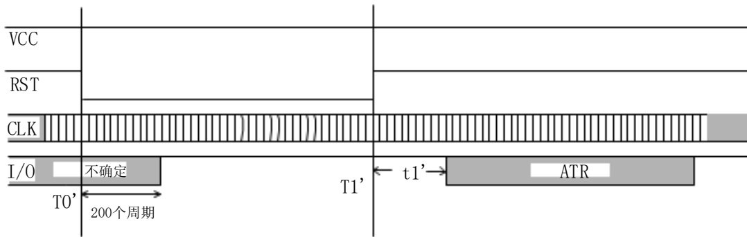
图8 热复位时序
