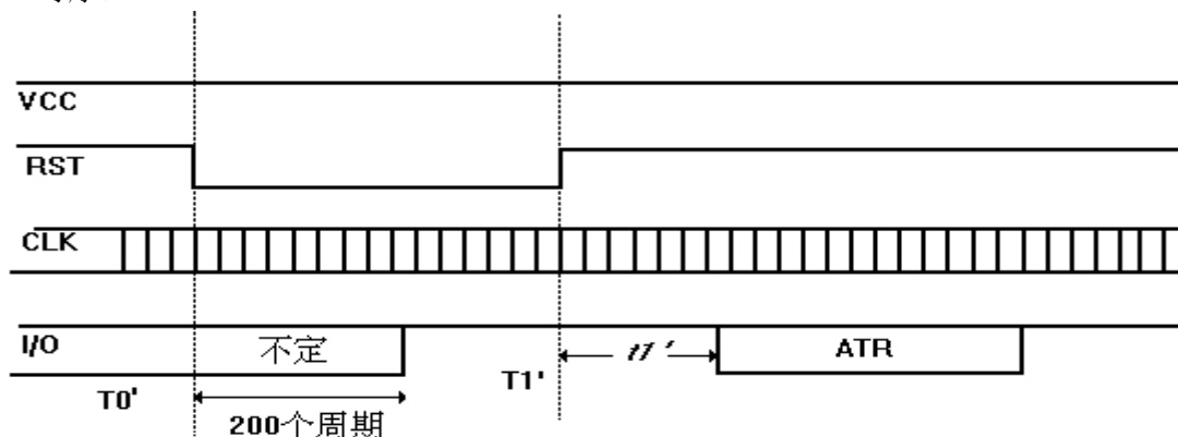
图8 热复位时序
