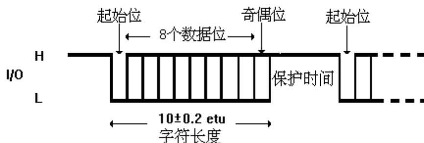
图10 字符帧
