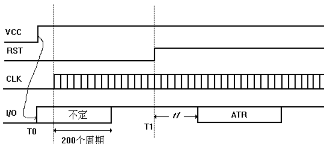
图7 冷复位时序
