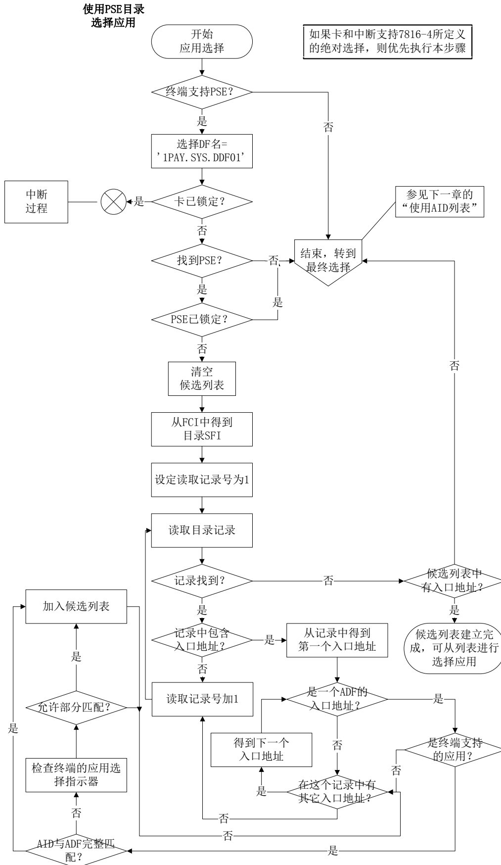
图15 使用目录方法的终端逻辑
