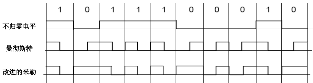
图3 编码图解
