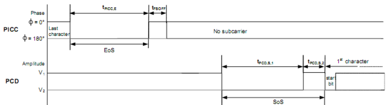
图9 PCD 的开始序列
