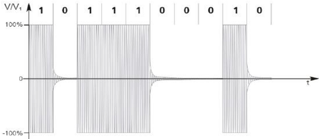
图2 OOK 编码
