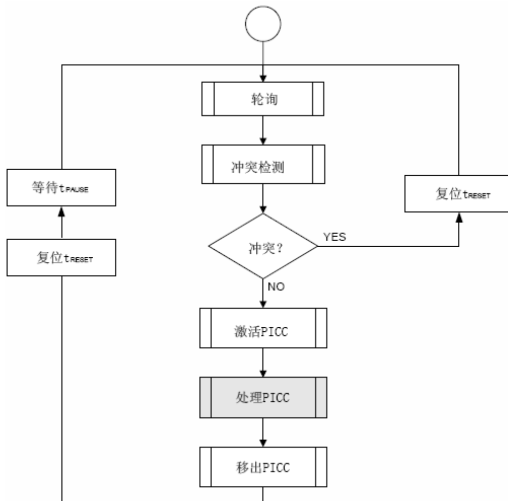
图25 终端主循环
