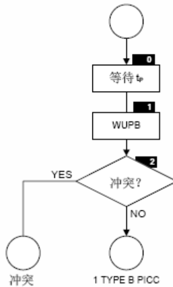
图28 Type B 冲突检测
