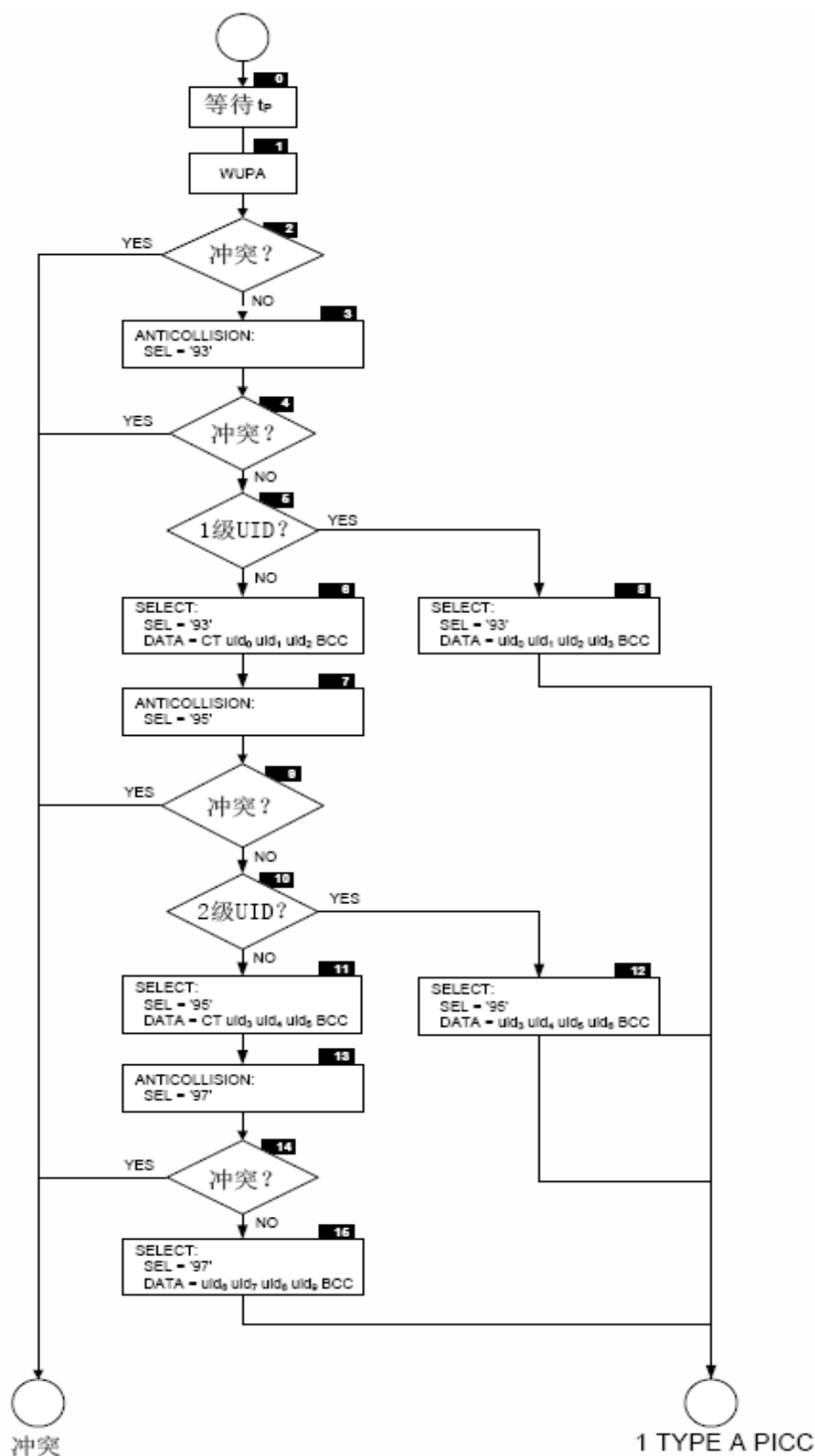
图27 Type A 冲突检测
