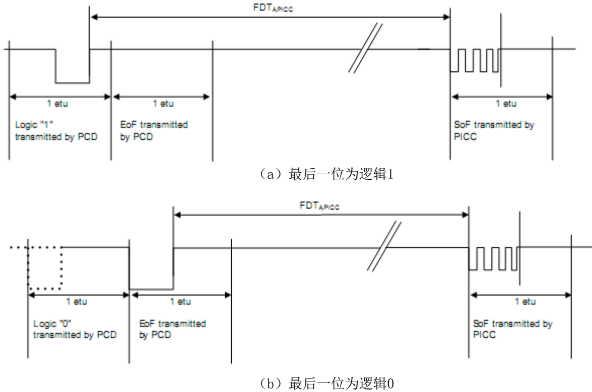
图15 FDT_{A,PICC}
