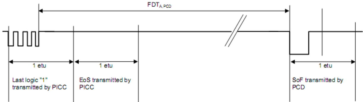
(a) 最后一位为逻辑 1
