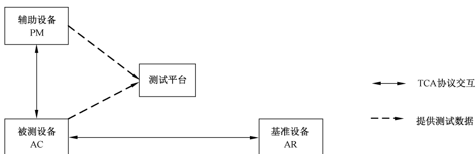
图 2 AC 测试拓扑
