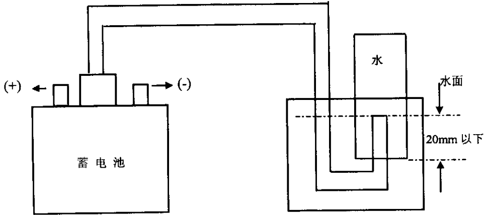
图3 收集气体示意
