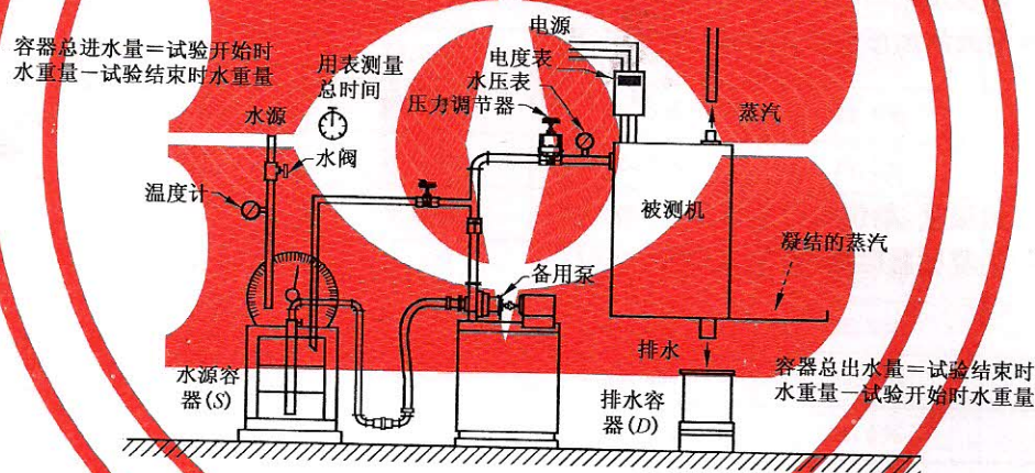
图 A.1 加湿量试验装置
