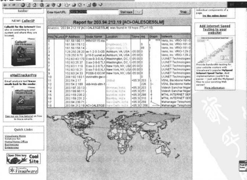
图 2-6 VisualRoute
