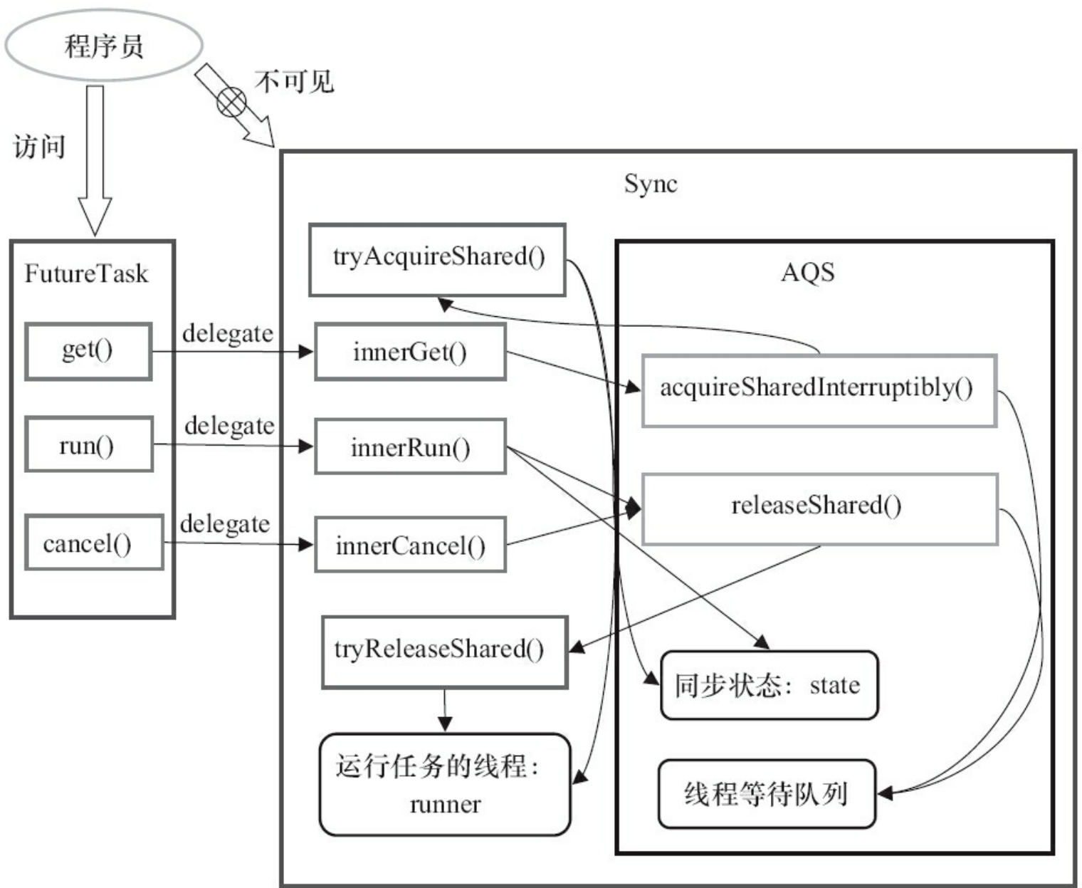
图10-15 FutureTask的设计示意图
