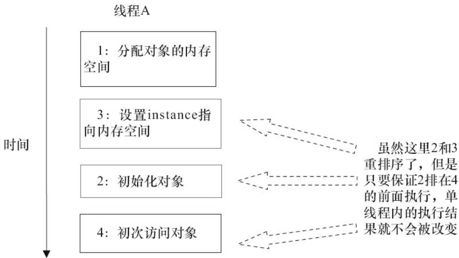
图3-37 线程执行时序图
