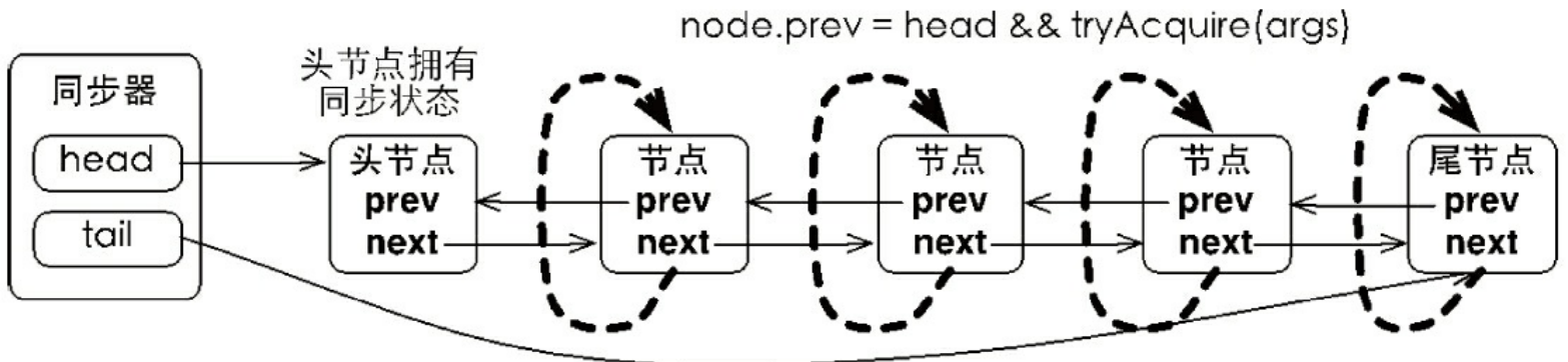
图5-4 节点自旋获取同步状态
