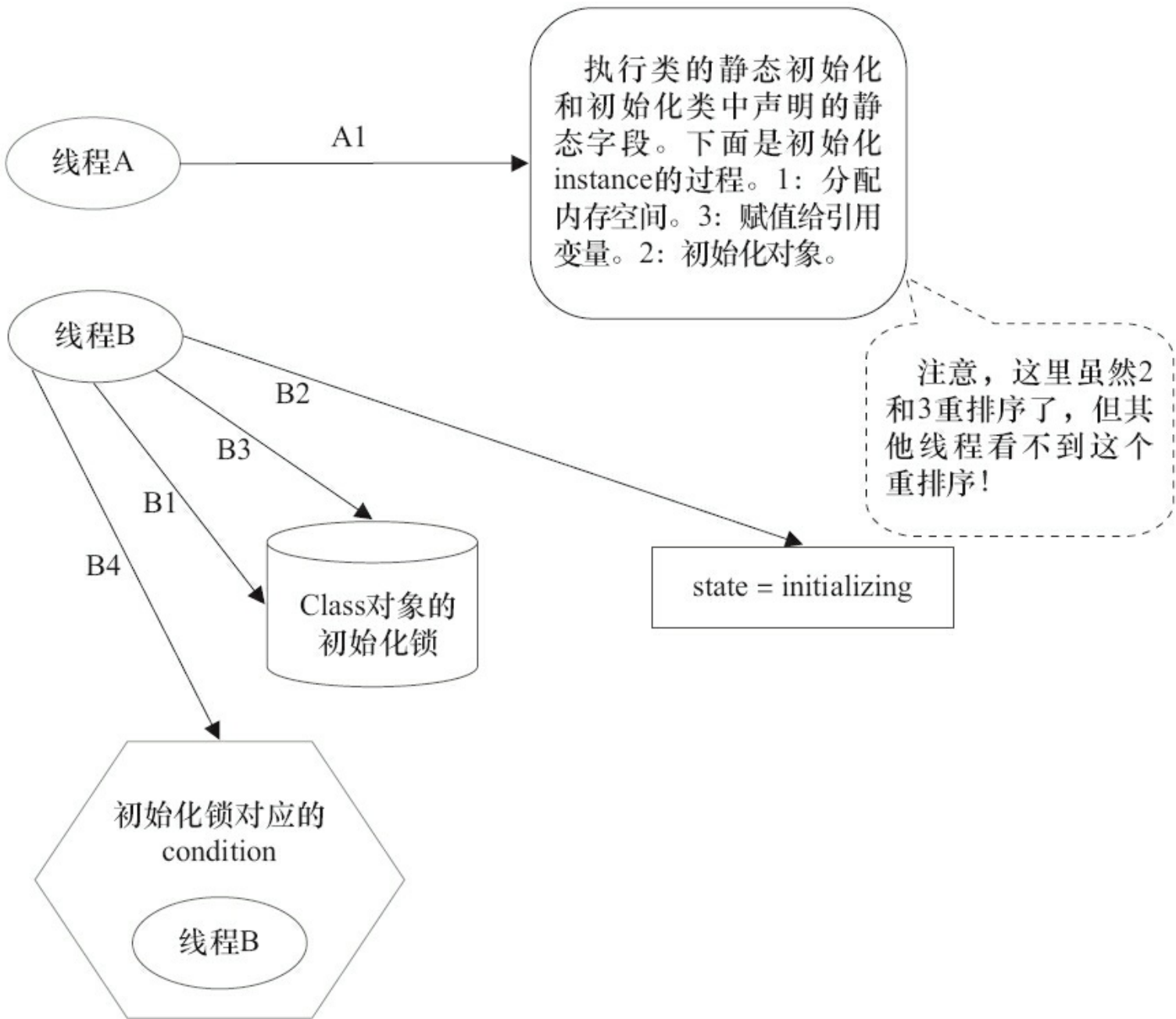
图3-42 类初始化——第2阶段
