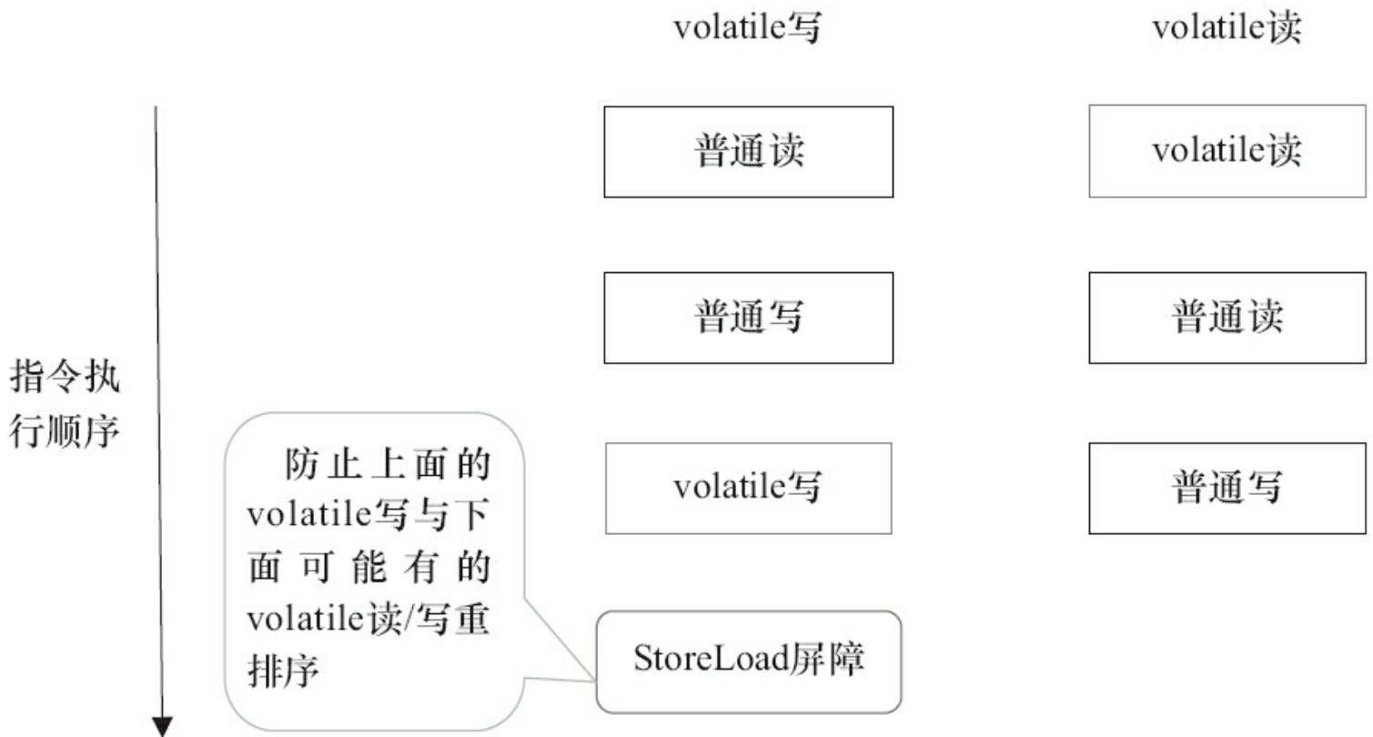
图3-22 指令序列示意图
