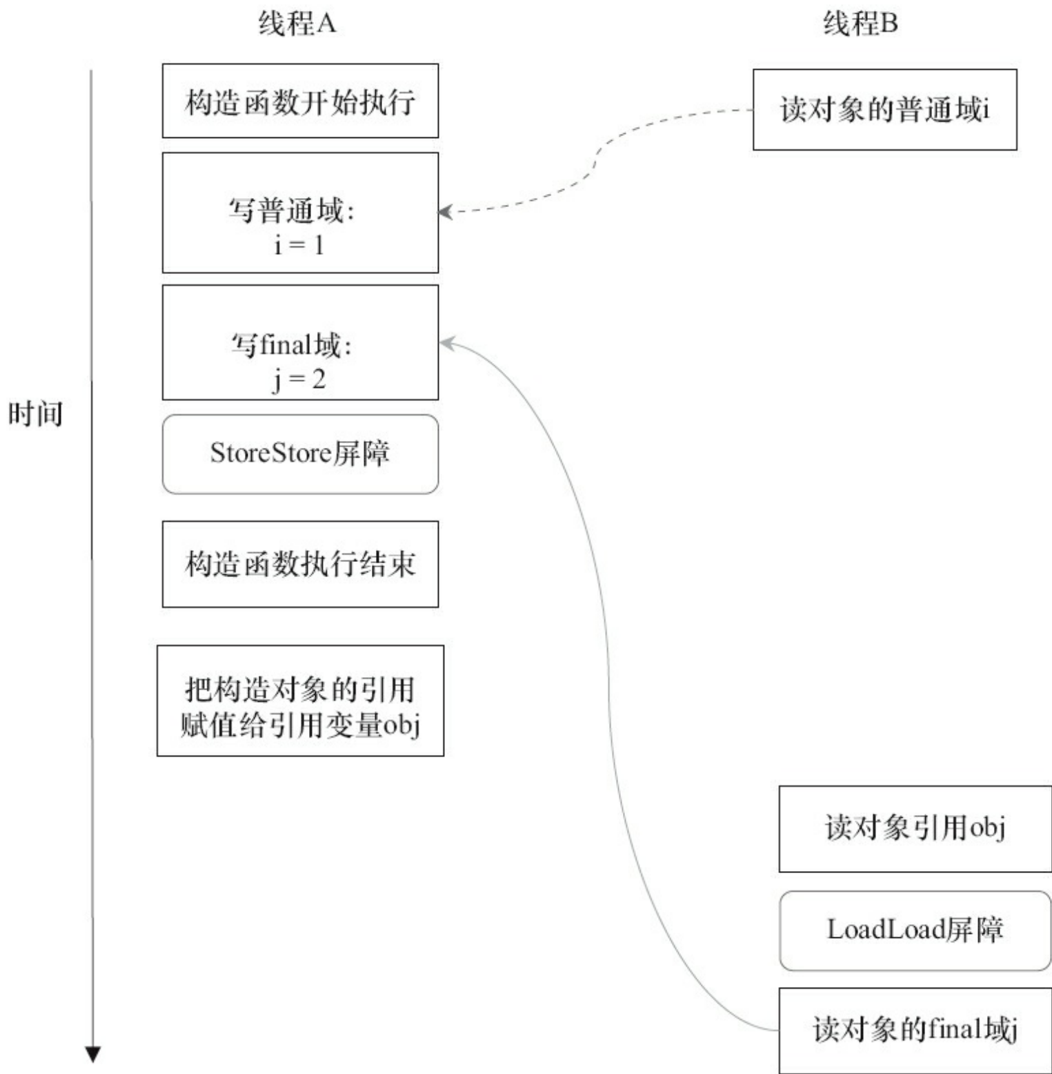
图3-30 线程执行时序图
