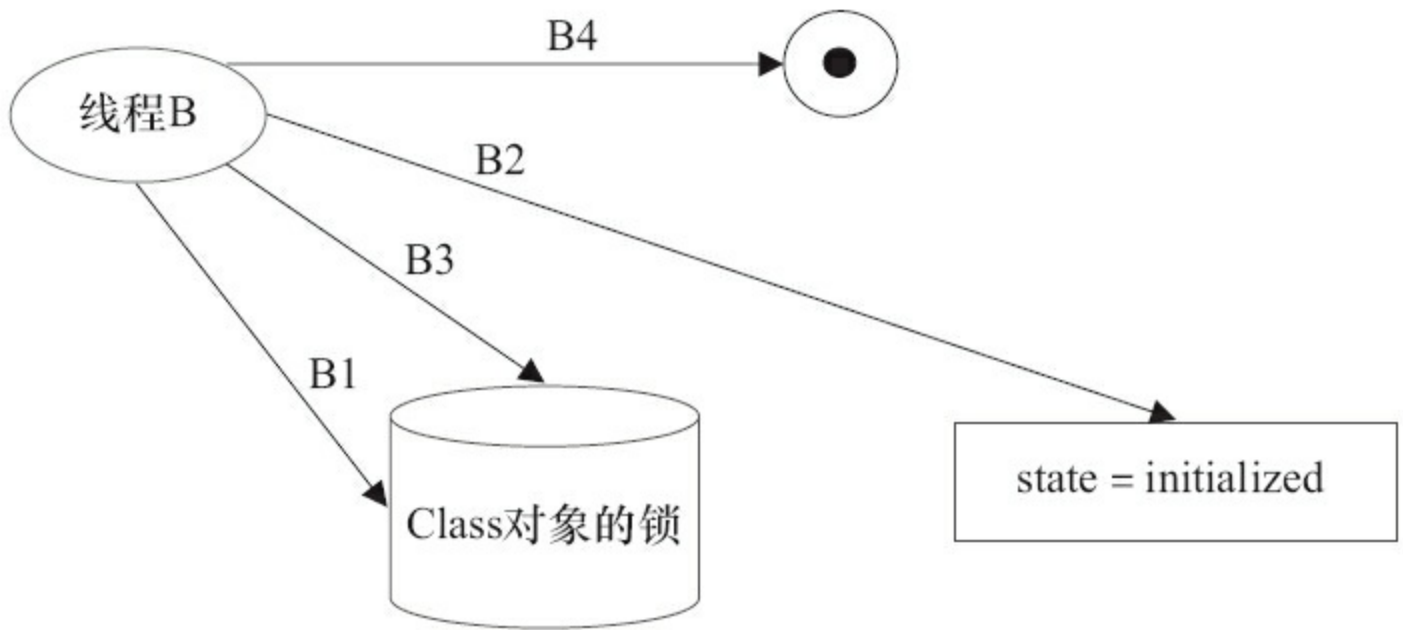
图3-44 类初始化——第4阶段
