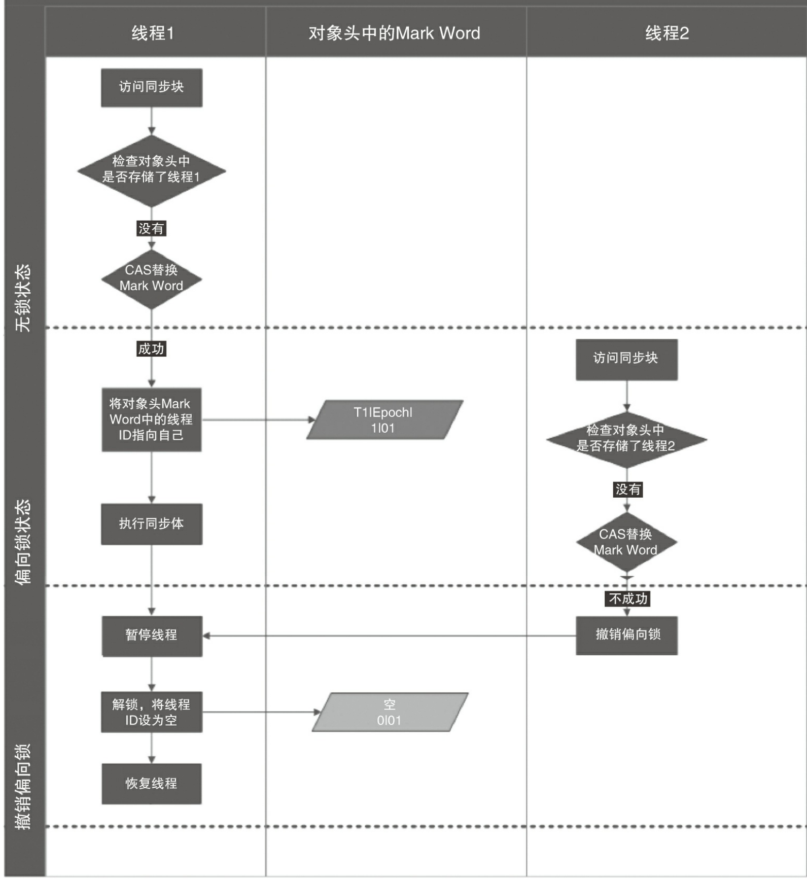
图2-1 偏向锁初始化的流程
