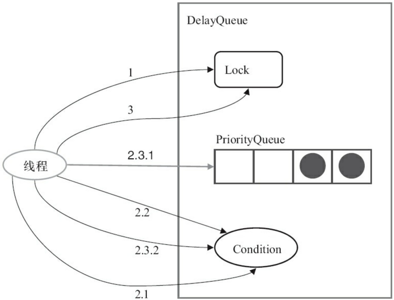
图10-10 ScheduledThreadPoolExecutor获取任务的过程
