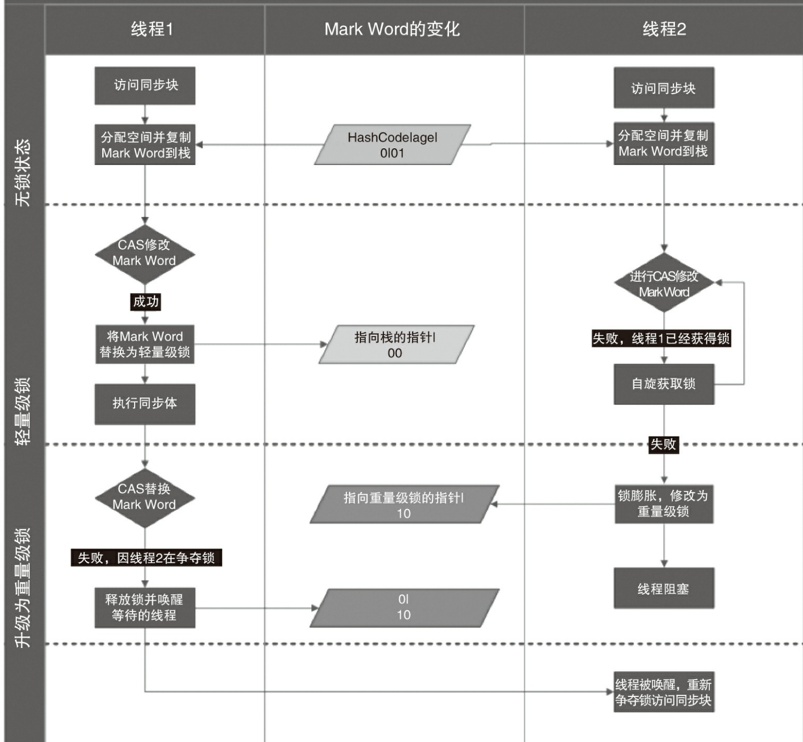
图2-2 争夺锁导致的锁膨胀流程图
