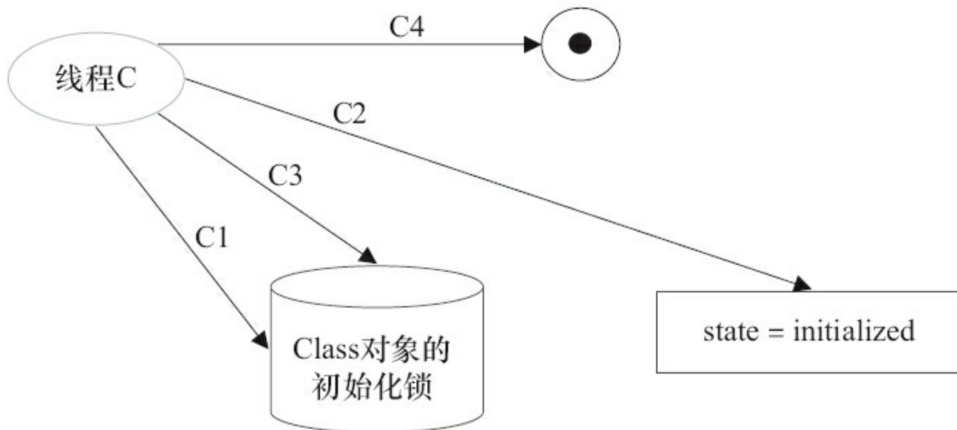
图3-46 类初始化——第5阶段
