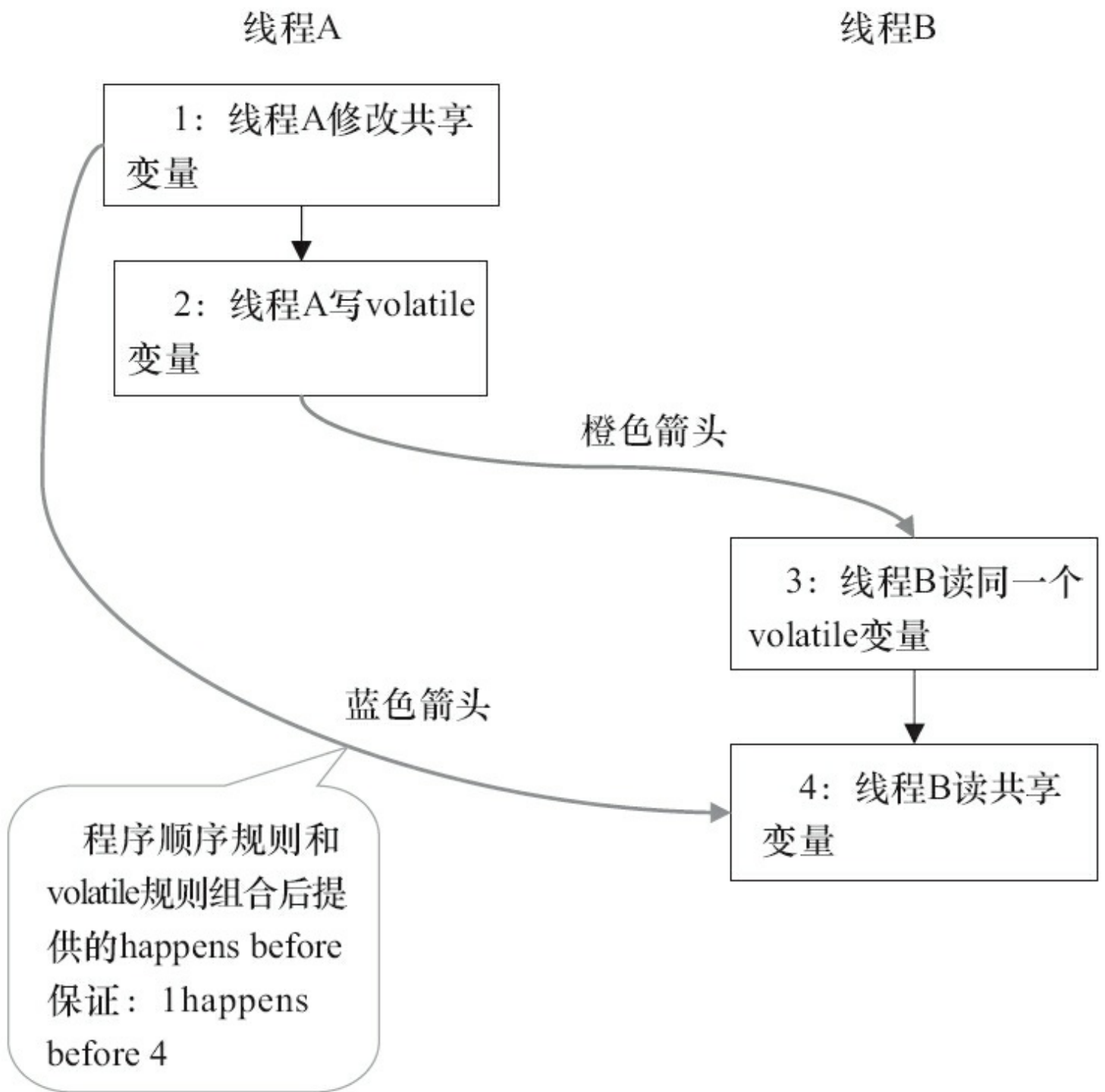
图3-16 happens-before关系
