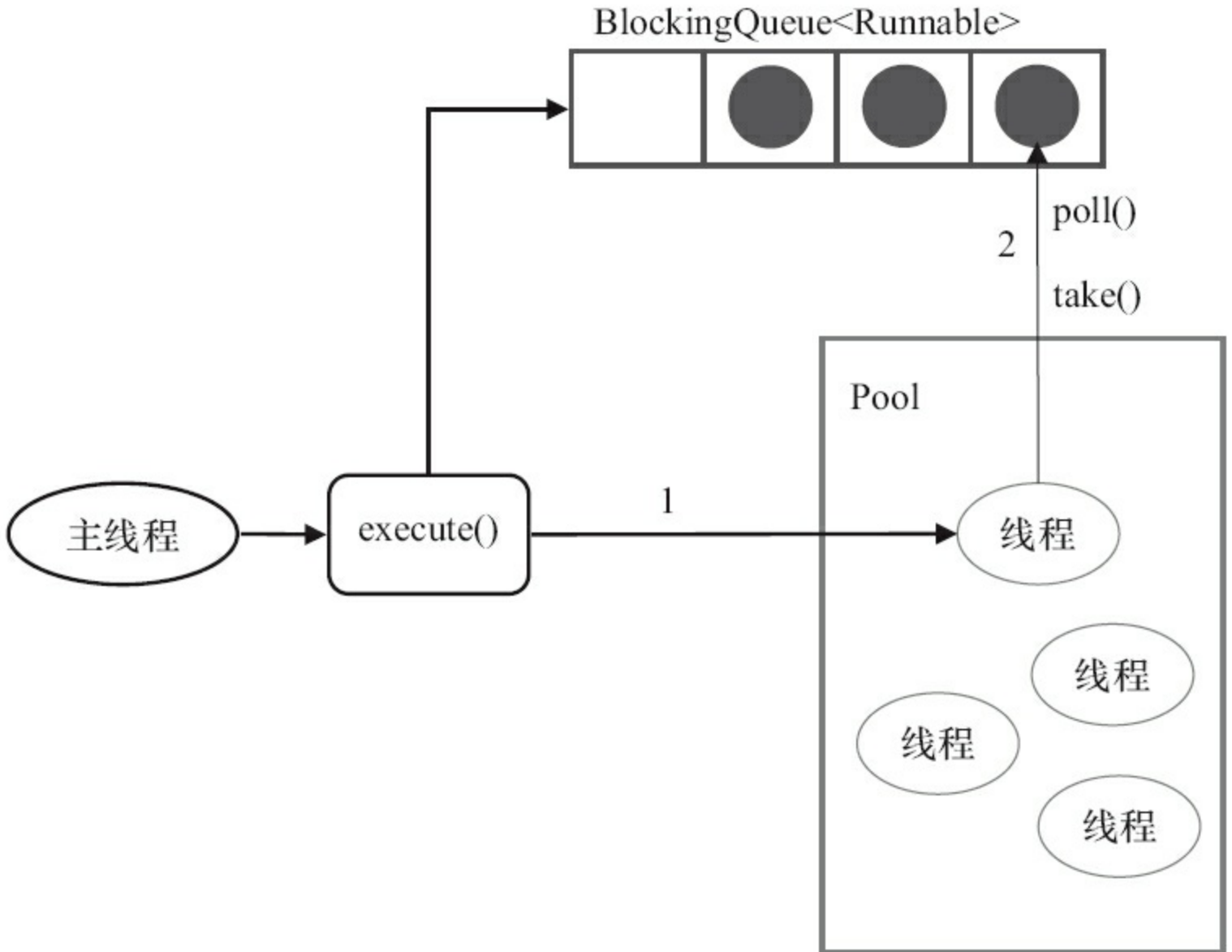
图9-3 ThreadPoolExecutor执行任务示意图
