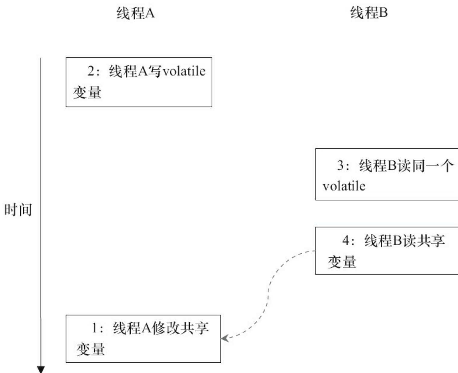
图3-23 线程执行时序图
