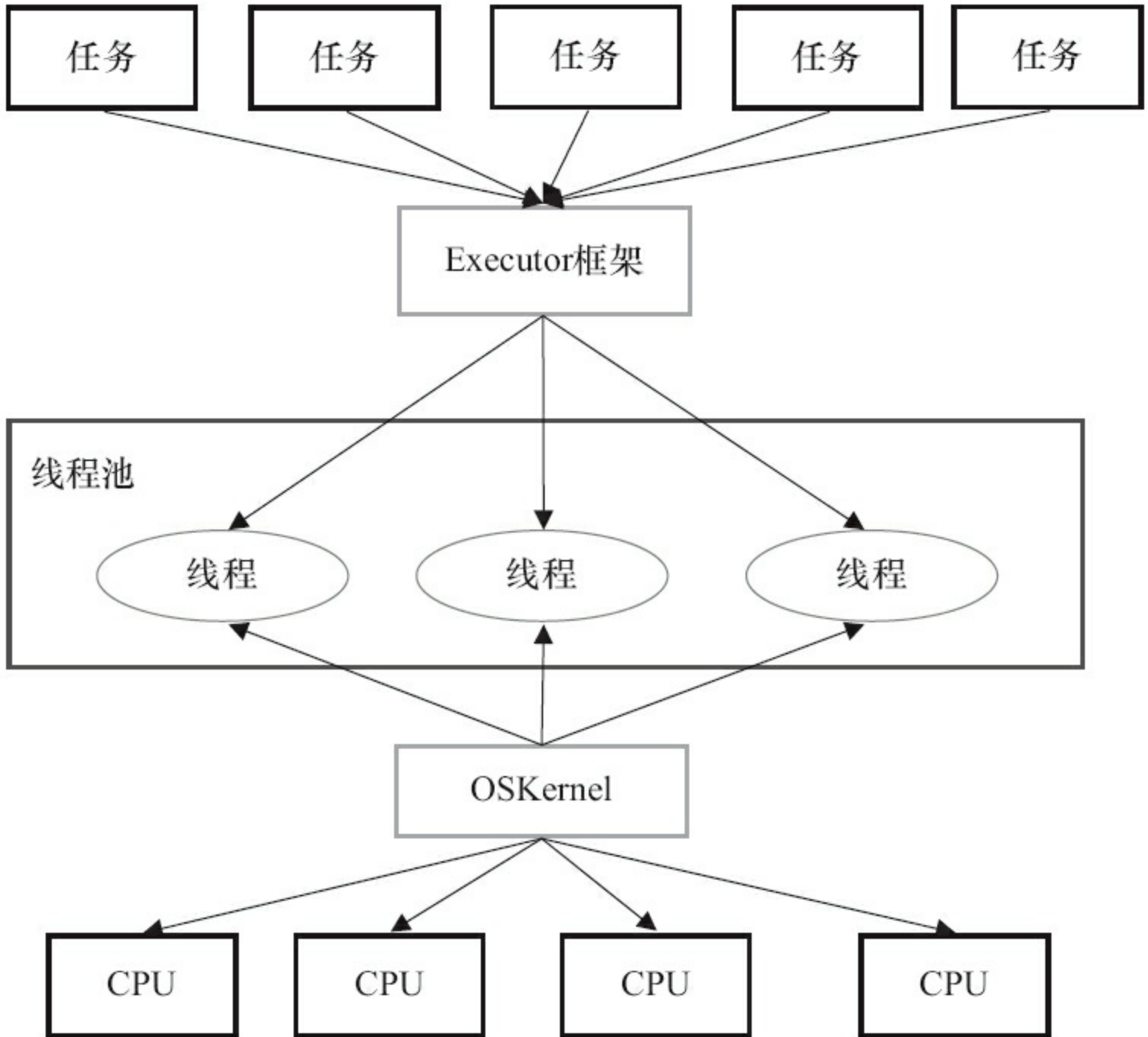
图10-1 任务的两级调度模型
