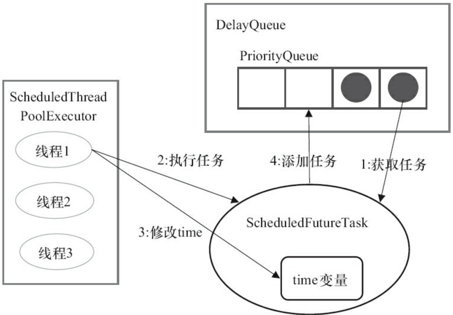
图10-9 ScheduledThreadPoolExecutor 的任务执行步骤
