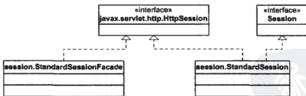
图 9-1 Session 管理相关类的 UML 类图
