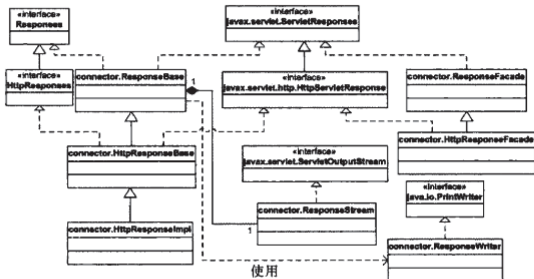
图 4-3 Response 接口及其相关实现类的 UML 类图
