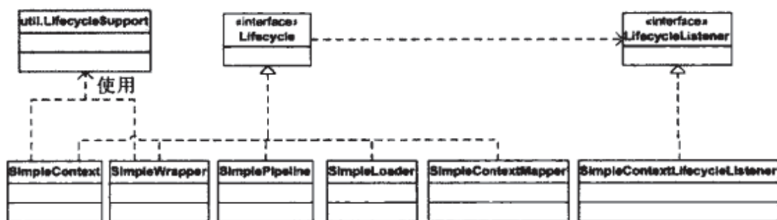
图 6-1 应用程序相关类的类图
