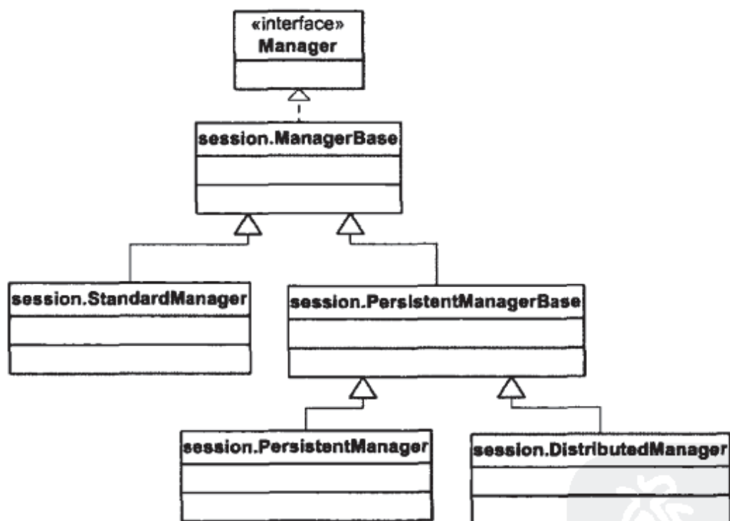
图 9-2 Manager 接口及其相关类的 UML 类图
