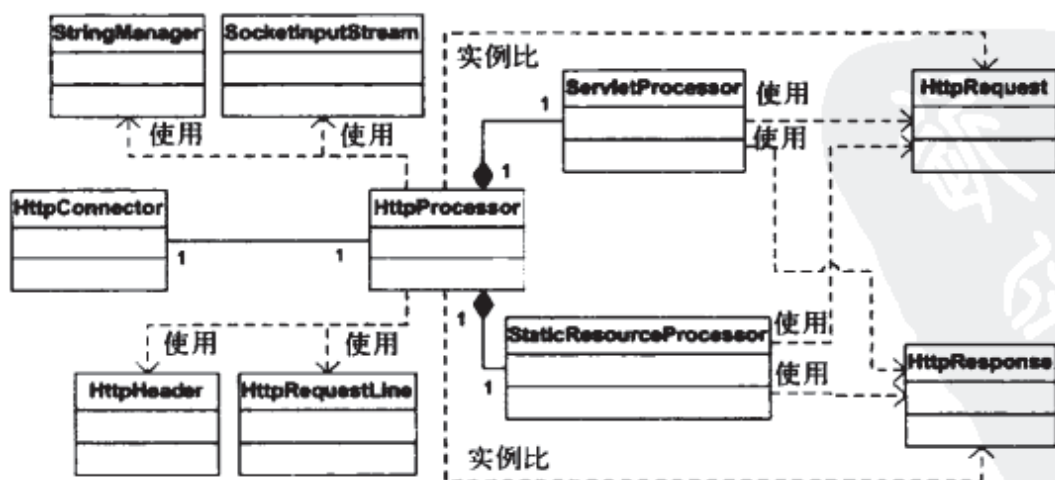
图 3-1 本章应用程序的 UML 类图
