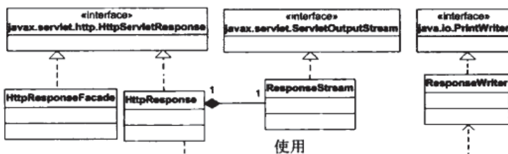
图 3-3 HttpResponse 及其相关类的 UML 类图
