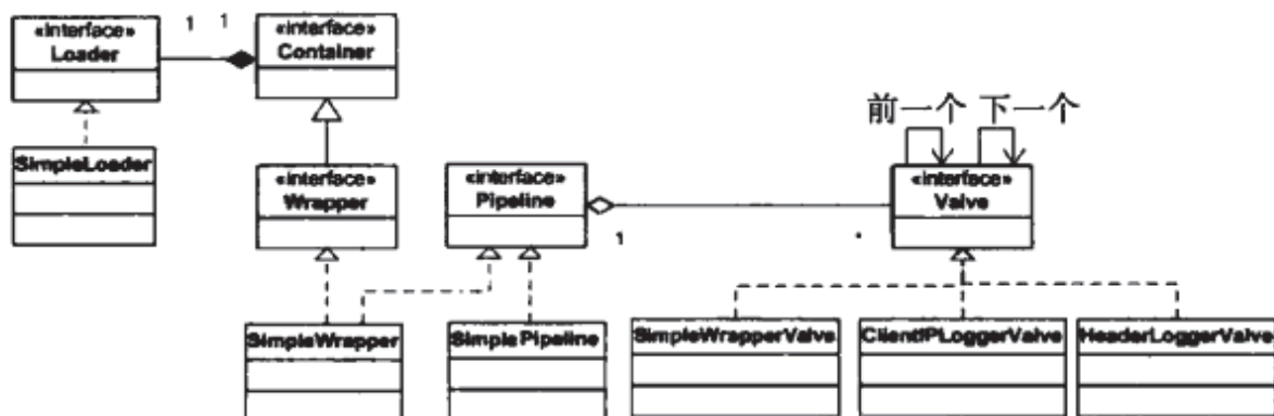
图 5-3 Wrapper 应用程序的 UML 类图
