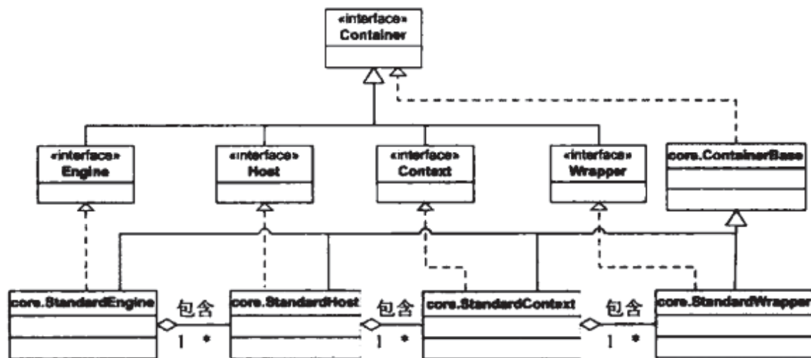
图 5-1 Container 接口及其相关类的 UML 类图
