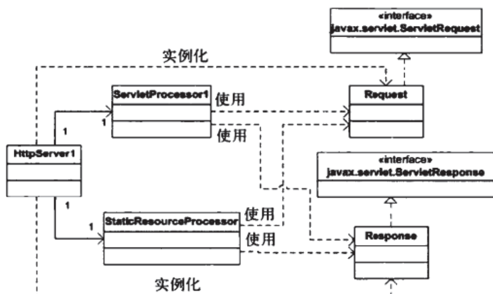
图 2-1 第一个 servlet 容器的 UML 类图
