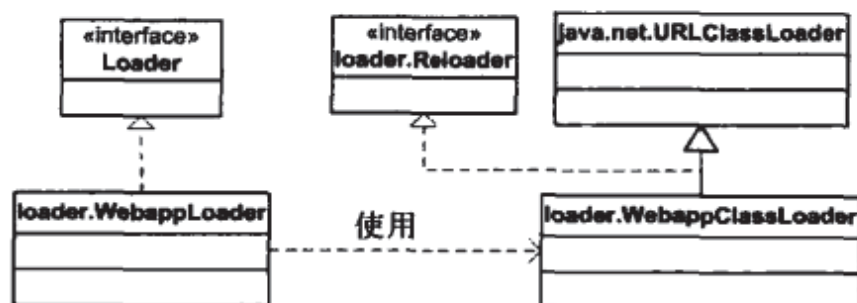
图 8-1 Loader 接口及其实现类的 UML 类图
