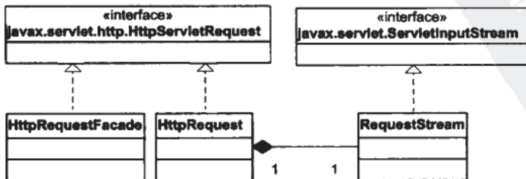
图 3-2 HttpRequest 类及其相关类的 UML 类图
