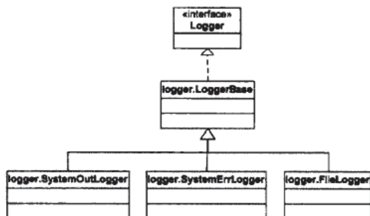
图 7-1 Tomcat 中的日志记录器相关类的 UML 类图
