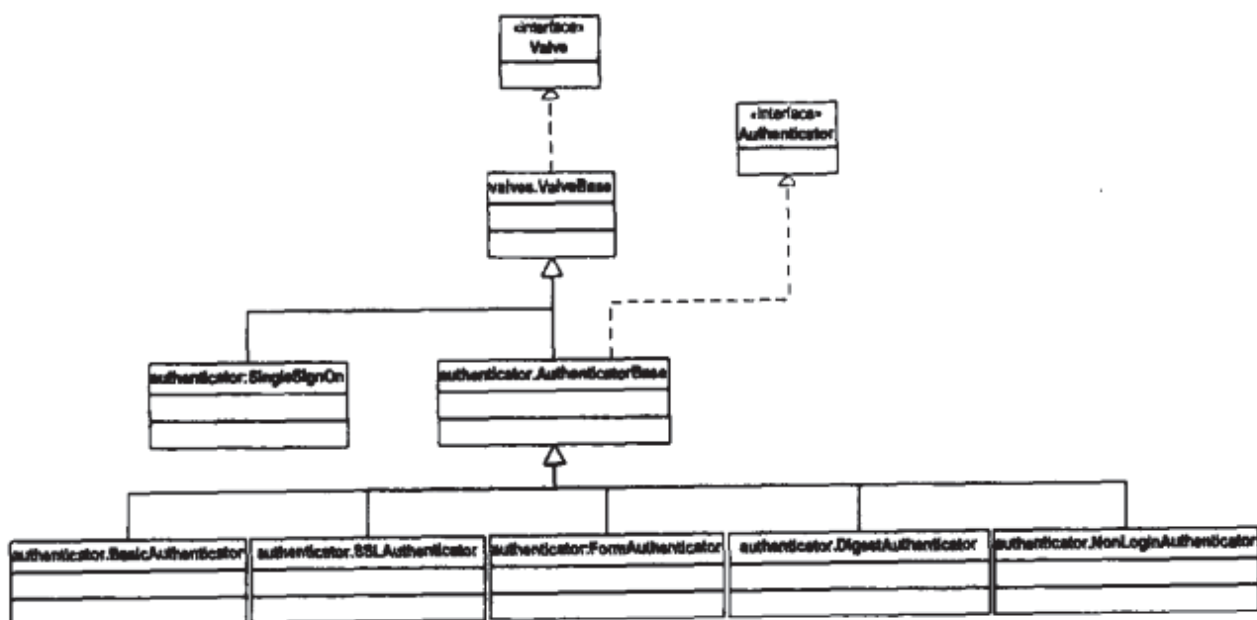
图 10-2 验证器相关类的 UML 类图
