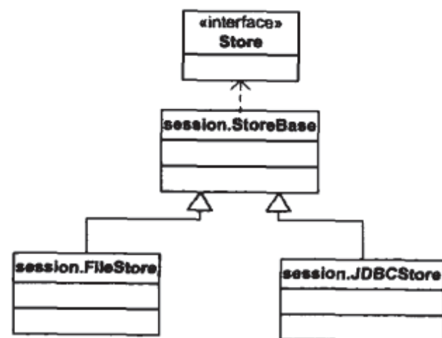
图 9-3 Store 接口及实现类的 UML 类图
