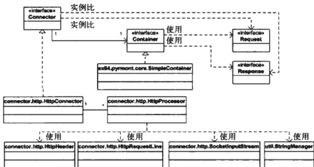
图 4-1 默认连接器的 UML 类图
