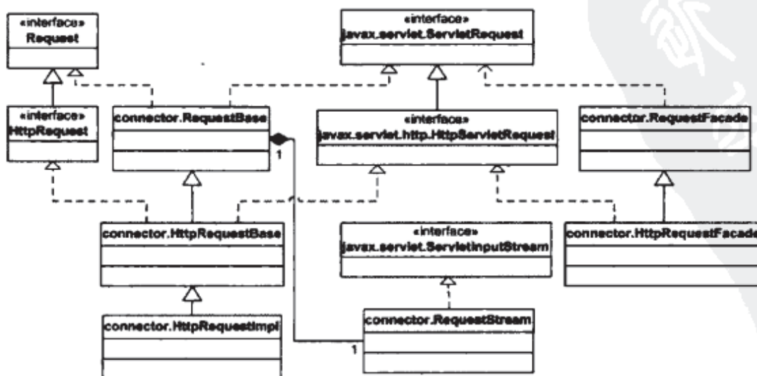
图 4-2 Request 接口及相关实现类的 UML 类图
