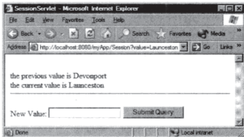
图 9-4 SessionServlet 类的输出
