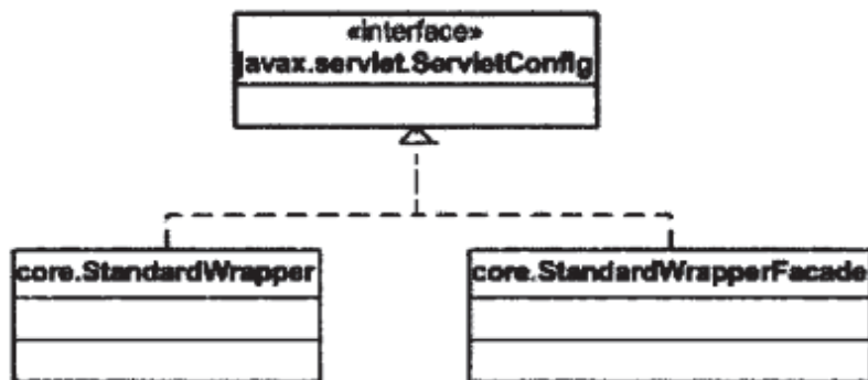
图 11-2 StandardWrapper 类与 StandardWrapperFacade 类之间的关系示意图
