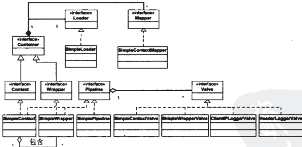
图 5-4 Context 应用程序相关类的 UML 类图
