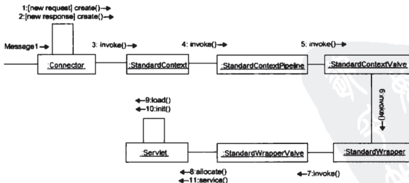
图 11-1 处理 HTTP 请求的方法调用协作图
