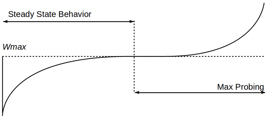
图 6.2: Cubic 函数
